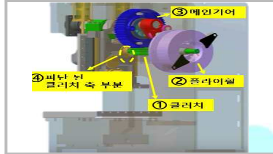
<구동부 구조>
